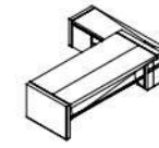
EUN-01D20-1 左 / 右班台 规格 (长W*宽D*高H) 2000W*1780D*760H
