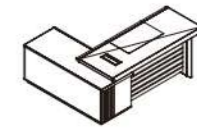
AXY-D0120 班台 2000 规格 (长W*宽D*高H) 2000W*1650D*760H
