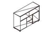
BG-S0312 文件柜 规格 (长W*宽D*高H) 1200W*400D*830H
