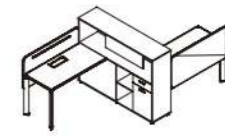
BG-D1528 两人位 规格 (长W*宽D*高H) 2800W*1600D*1200H
