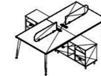
名称 Name ASY-D0524 职员位 规格 Size 2430W×2400D×750H
