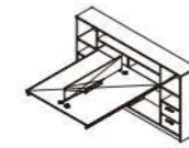
BG-D1716YS 两人位 (延伸) 规格 (长W*宽D*高H) 1660W*2000D*1100H
