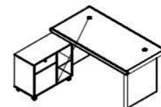
名称 Name ASY-02D16 班台 规格 Size 1600W×800D×750H 活动柜 800W×400D×650H
